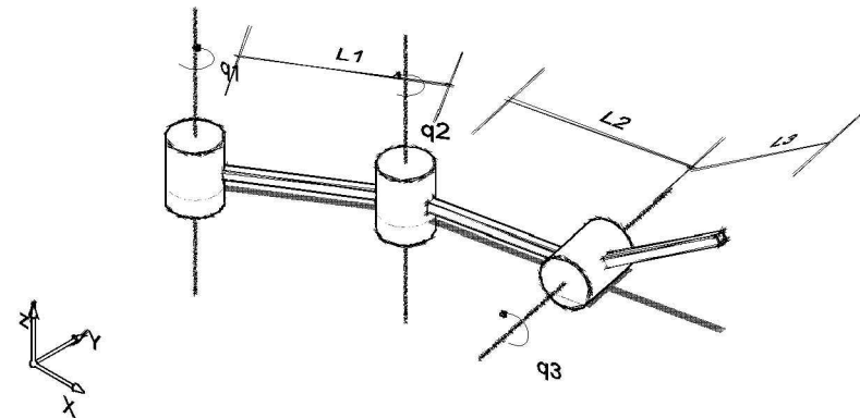
Vista Isométrica (ejemplo de movimiento)
